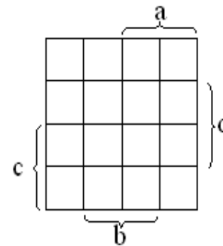
c) 4 variabili
