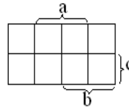
b) 3 variabili
